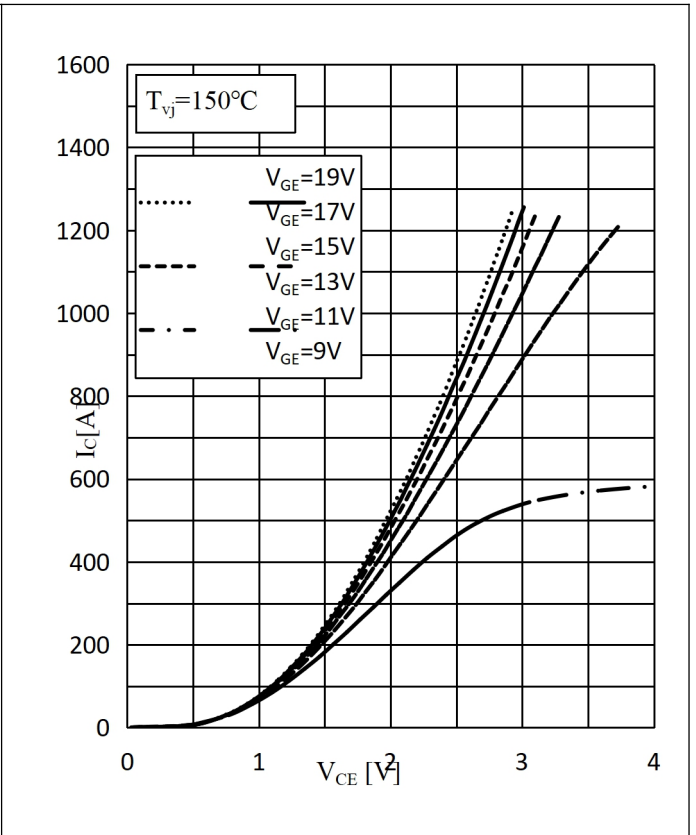
Fig.2: Output characteristics 图 2: 输出特性
