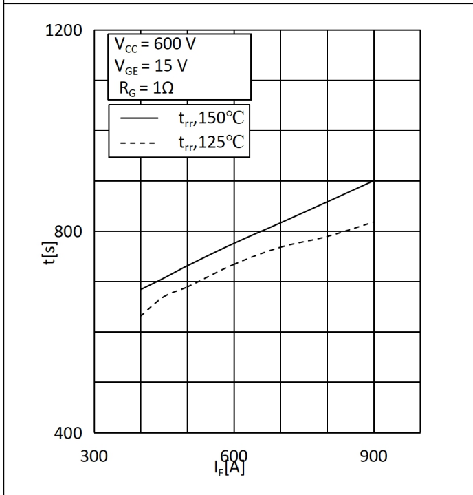
Fig.11: Reverse Recovery Times vs. I_F -Chopper 图 11: 反向恢复时间与正向电流关系-斩波
