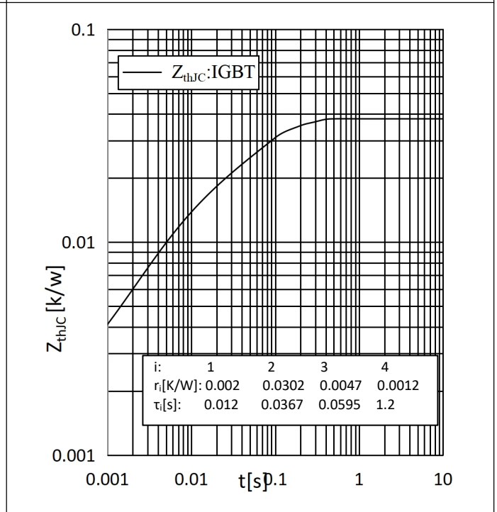
Fig.13: Typ. transient thermal impedance(IGBT) Z_{thJC} IGBT(K/W) 图 13: 典型的瞬态热阻抗(IGBT) Z_{thJC} IGBT(K/W)
