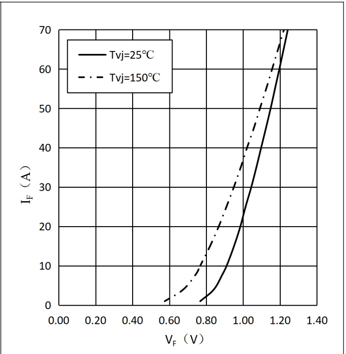
Fig.10 Forward Characteristics of Diode-Rectifier 图 10 二极管正向偏压特性-整流器
