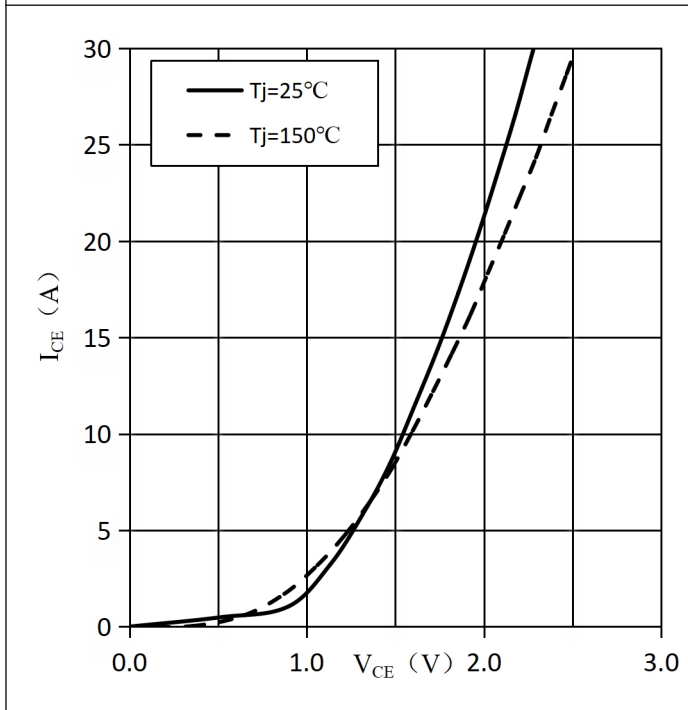
Fig.11 Typ. Output Characteristics, Brake-Chopper 图 11 输出特性, 制动-斩波器
